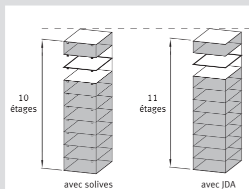
Hauteur de construction réduite avec les armatures anti-poinçonnement JORDAHL® JDA
